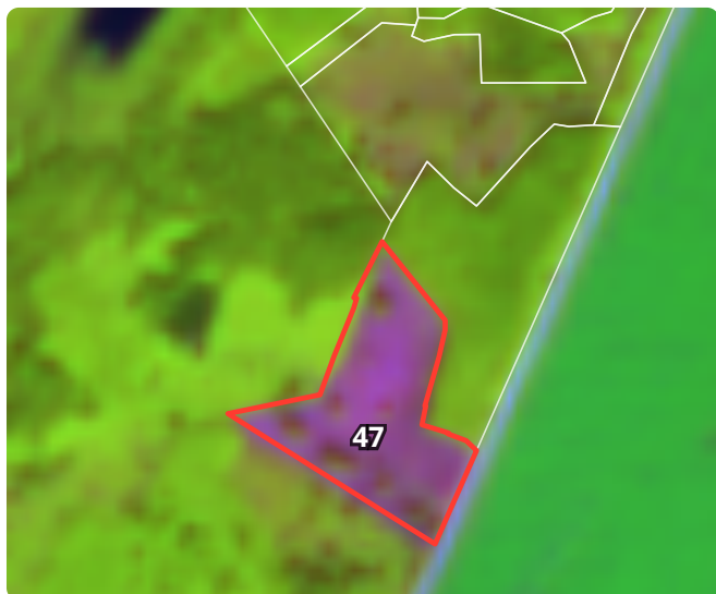
Pēc (infrasarkanā kanālī) · 20.06.2026: mežs zaļš, izcirtums violets vai sārts
